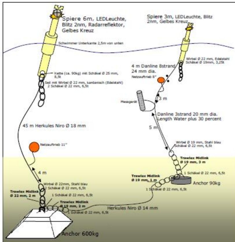
Abb. 3: Schematische Zeichnung des POD-Verankerungssystems von BioConsult SH.
